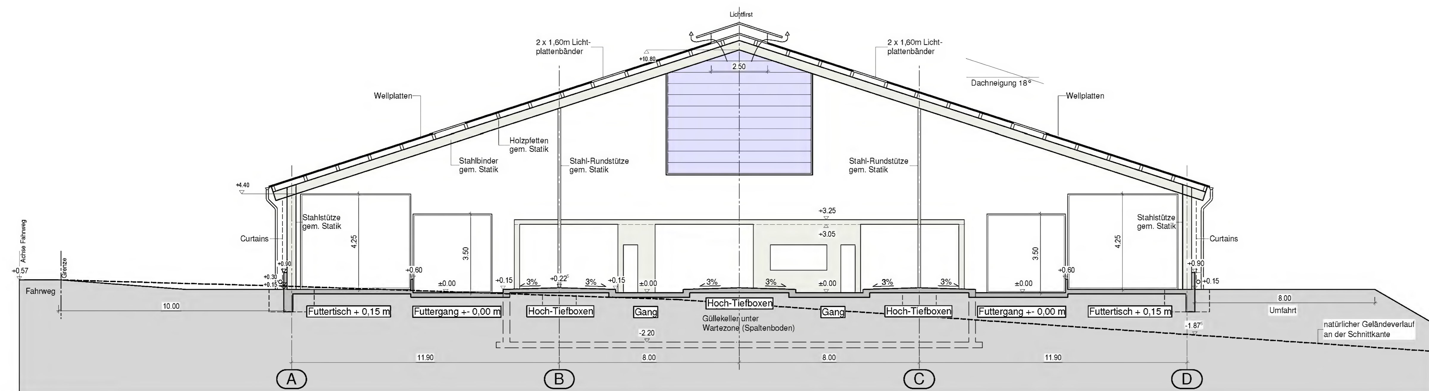
SCHNITT A-A
