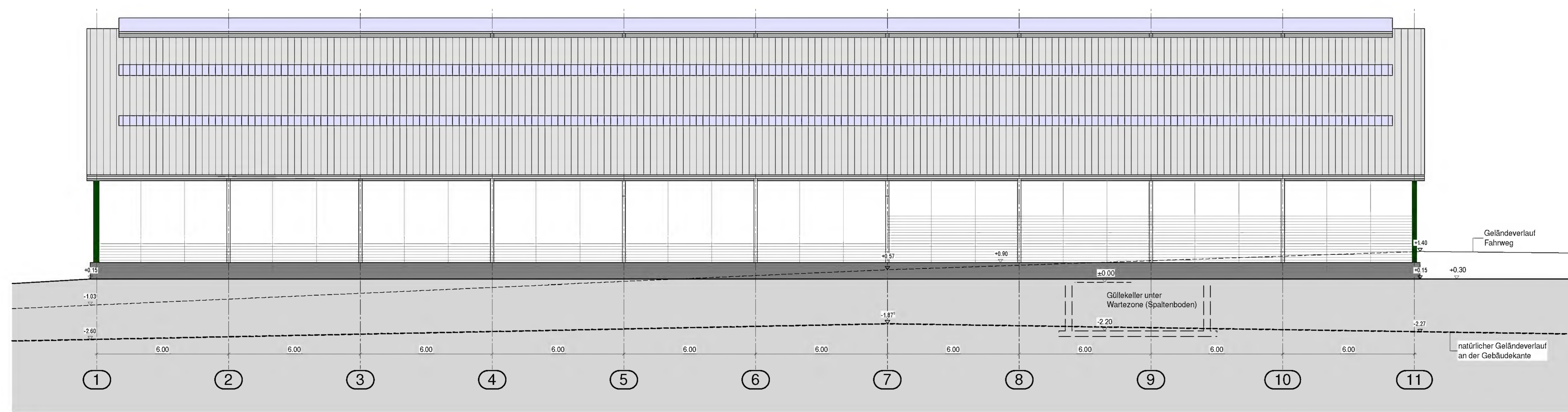
ANSICHT SÜD-WEST
